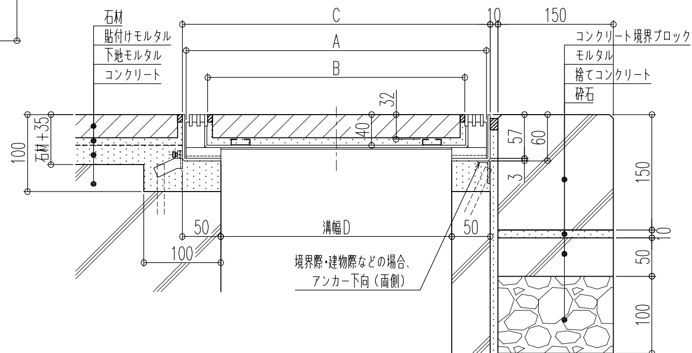
施工参考図
